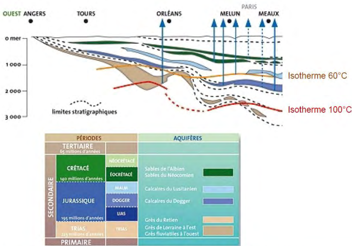
Illustration 11 : Coupe n° 2 nord-est - sud-ouest, puis est-ouest, en région Centre.
