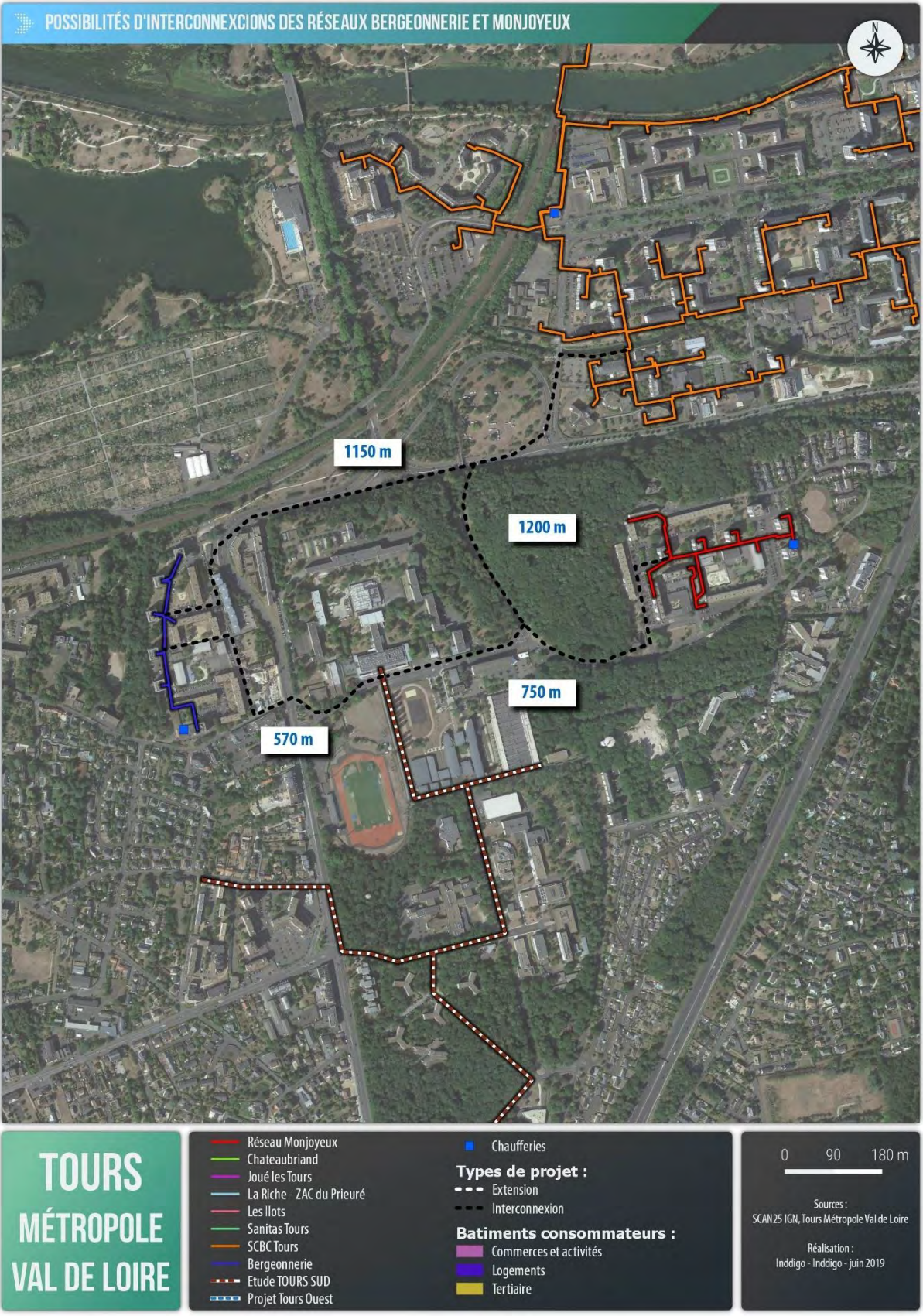
Figure 31 : Tracé des interconnexions potentielles vers Bergeonnerie et Montjoyeux
