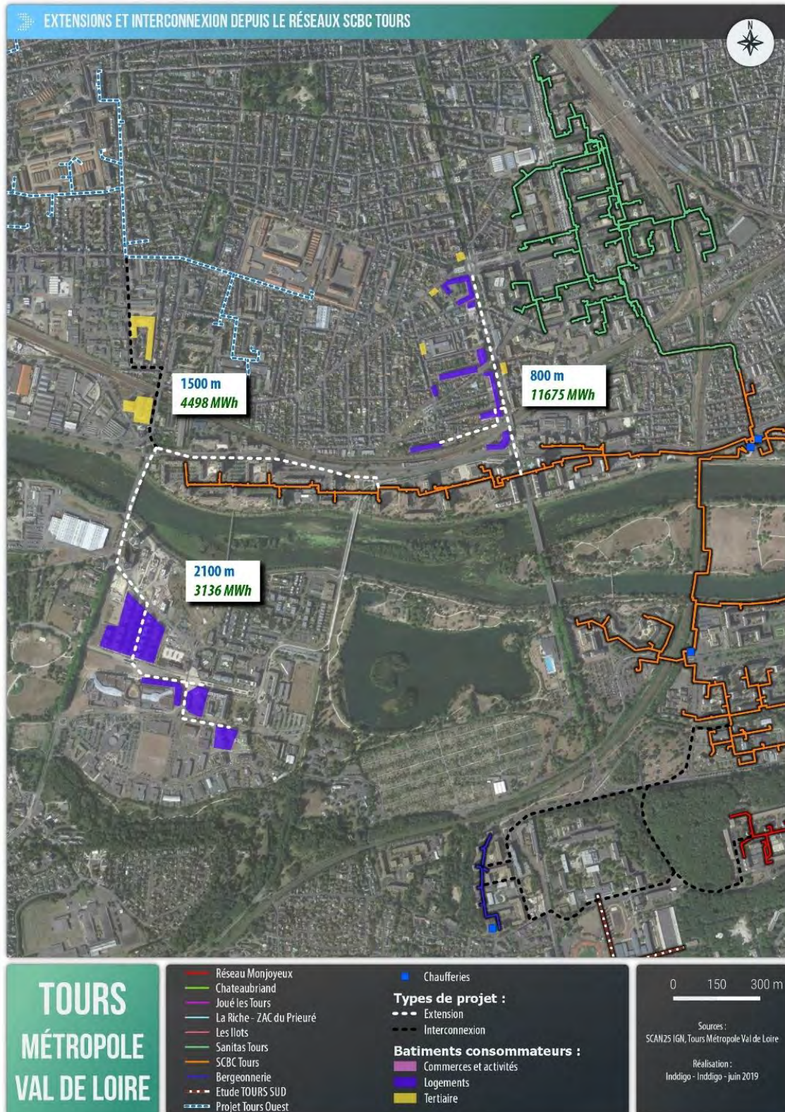
Figure 28 : réseau SCBC - opportunités d'extension
