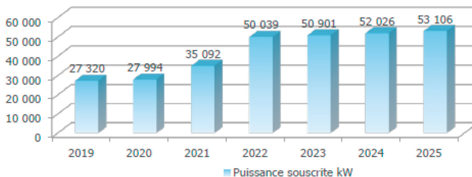
Figure 20 : Développement du réseau de chaleur en projet de 2019 à 2025 - Source Engie Cofely
