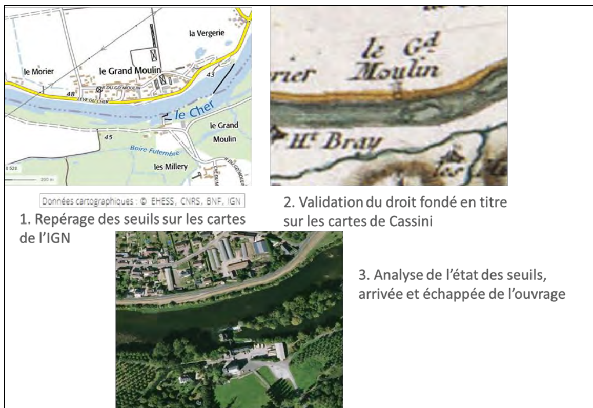
Figure 17 - Exemple des étapes de repérage d'un ouvrage: le Grand Moulin de Ballan Miré
