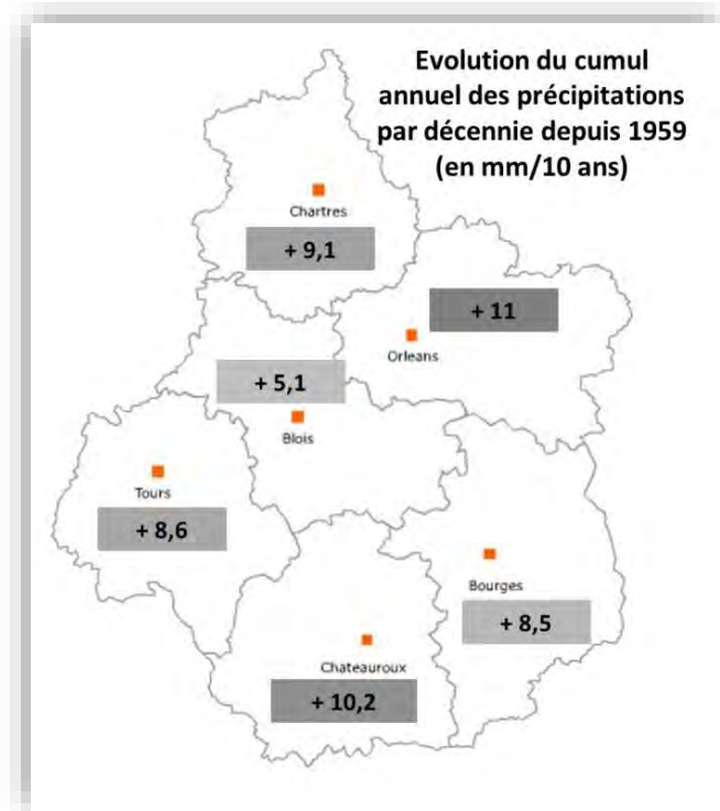
Figure 14 : Cumul annuel des précipitations par décennie (Chambre régionale d'agriculture CVL 2021, p 6)
