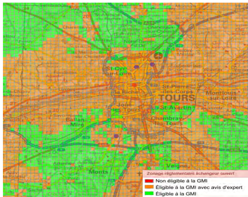
Figure 39 : Zones réglementaires GMI - Sur aquifère - Source Géothermie Perspectives (BRGM)
